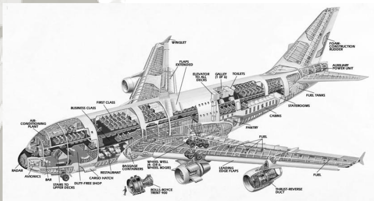
Airbus A380 felépítése
